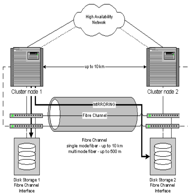
Рис. 1. Географически распределенный кластер
