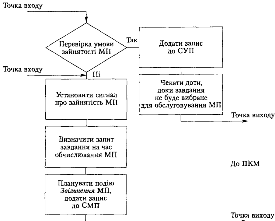
Рис. 5.11. Фрагмент блок-схеми призначення процесора завдання
