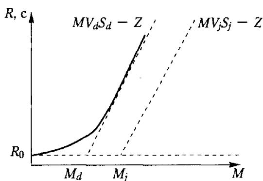
Рис. 2.22. Залежність часу перебування вимоги від кількості пристроїв у замкненій мережі
