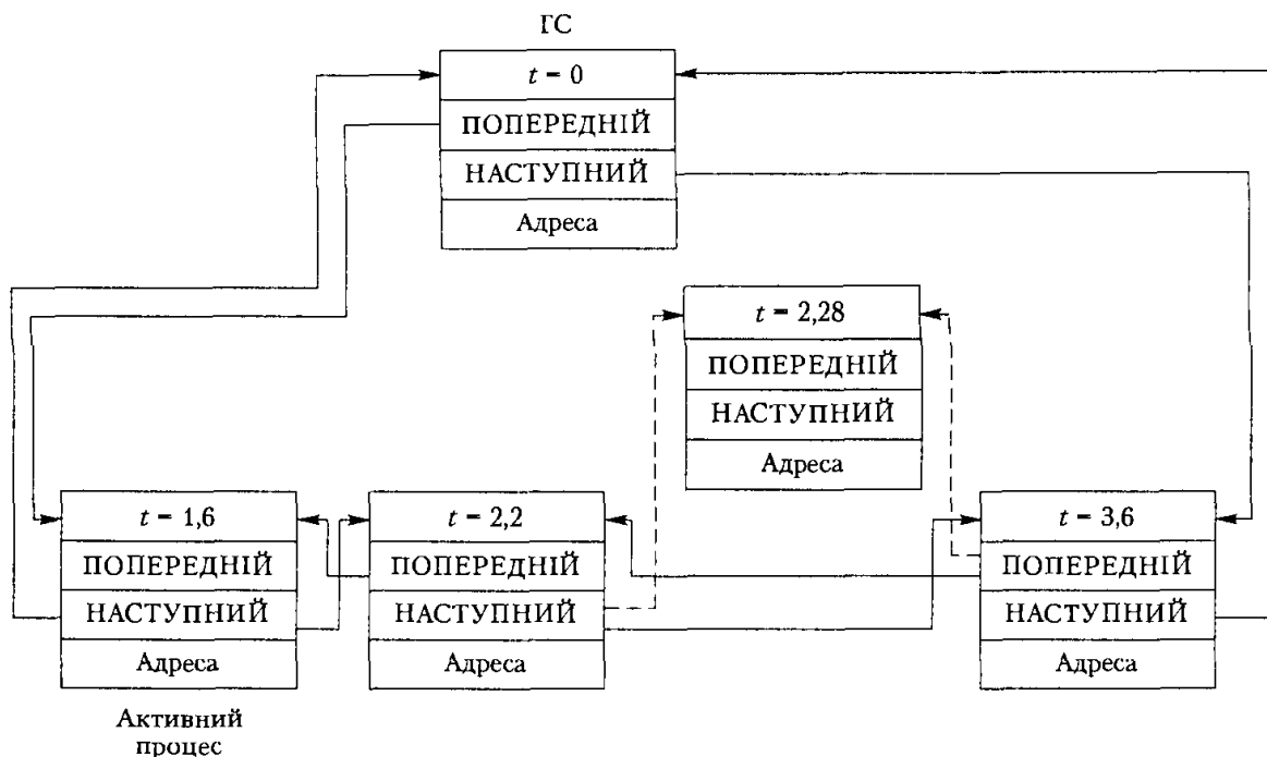
Рис. 6.4. Організація циклічного двонапрявленого списку
