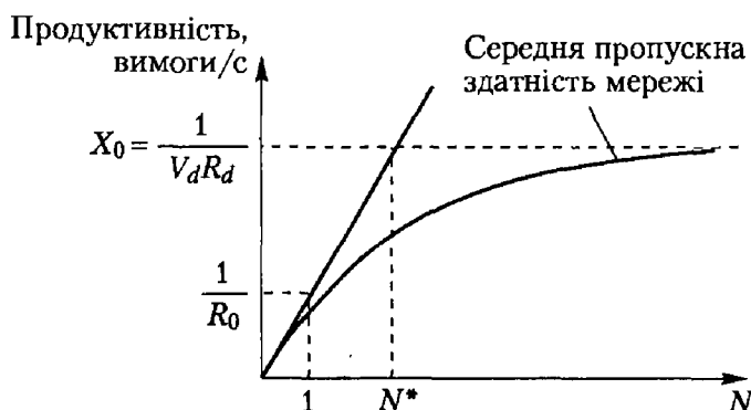
Рис. 2.21. Графік залежності продуктивності мережі від кількості вимог
