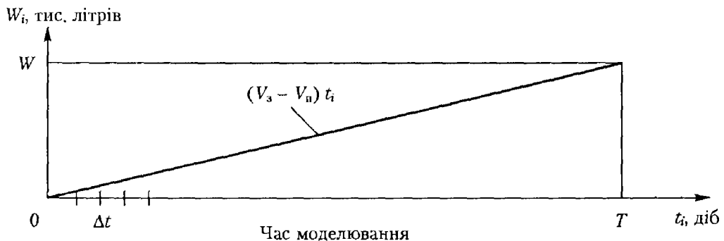
Рис. 1.5. Динамічна характеристика наповнення резервуара
