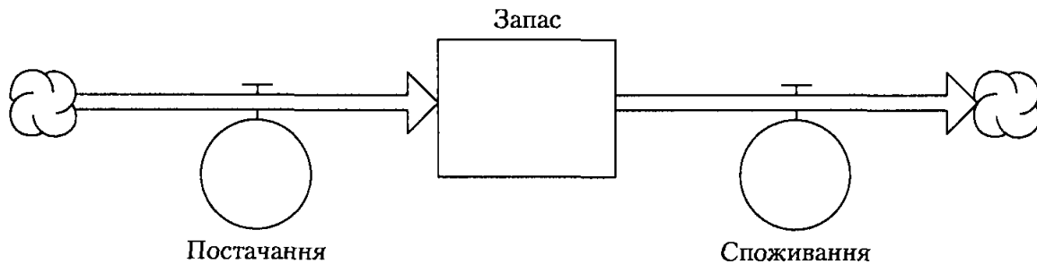
Рис. 6.7. Потокова модель
