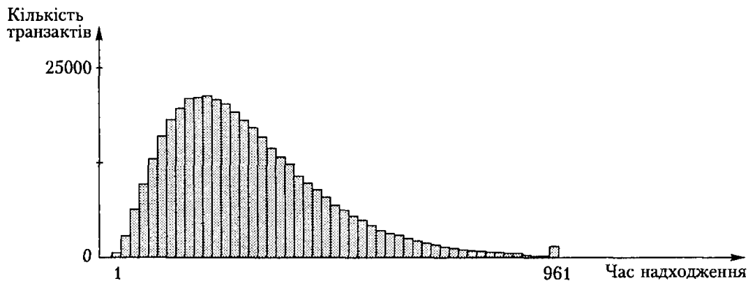
Рис. 4.19. Гістограма, отримана за результатами моделювання
