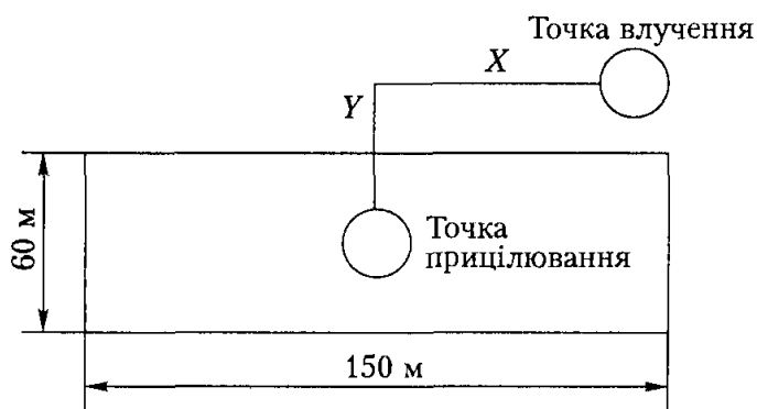
Рис. 4.29. Схема влучення ракети в ціль
