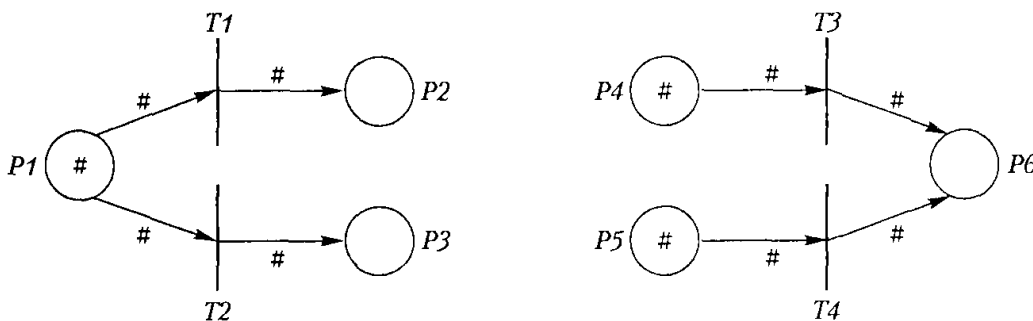
Рис. 3.21. Конкуруючі переходи
