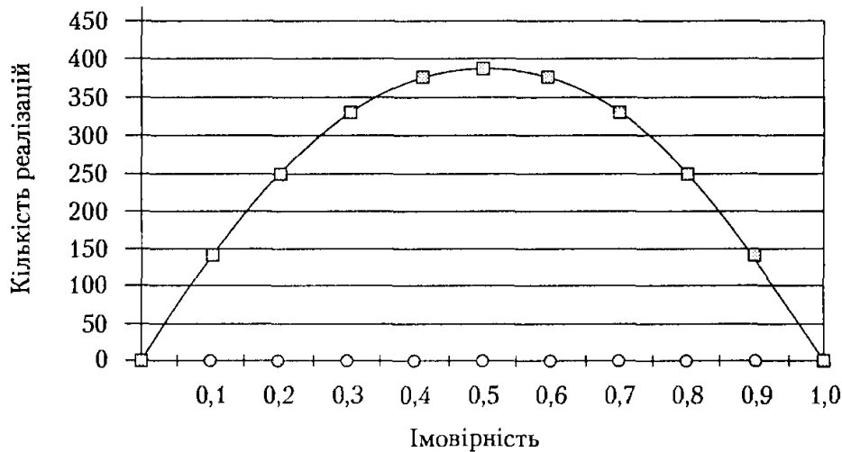
Рис. 4.28. Залежність числа реалізацій від значень ймовірності
