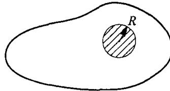
Рис. 4.2. Схематичне зображення враження цілі бомбою
