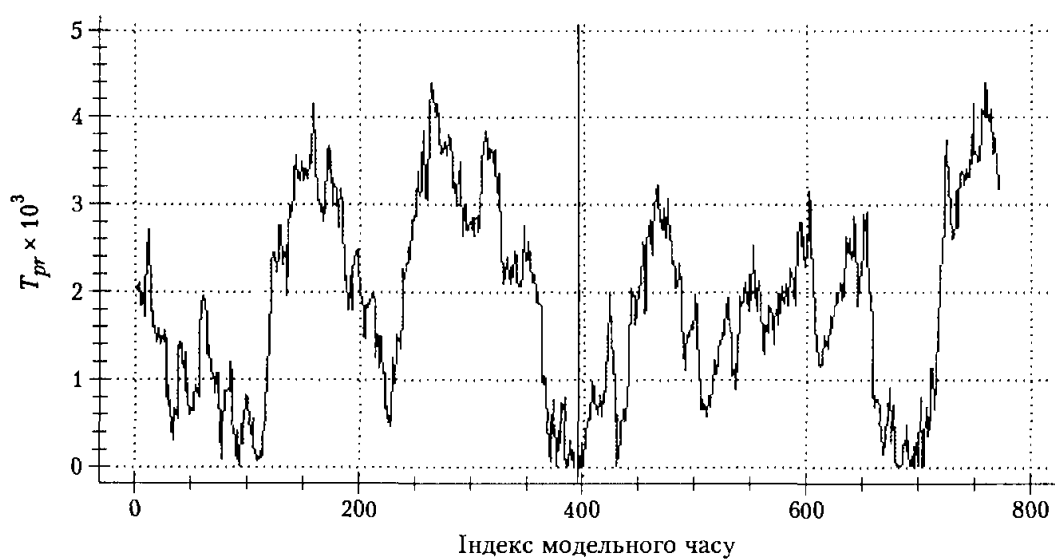
Рис. 7.18. Відновлений ряд
