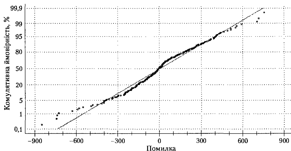
Рис. 7.16. Функція розподілу помилки моделювання
