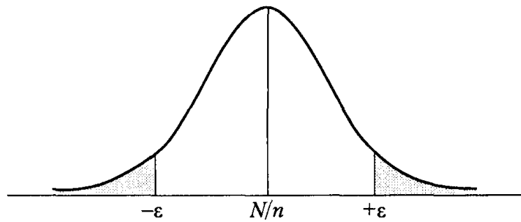
Рис. 4.27. Функція нормального розподілу для побудови довірчого інтервалу
