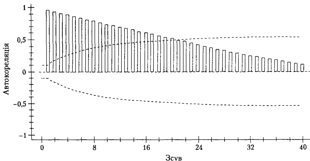
Рис. 7.14. Автокореляційна функція часового ряду
