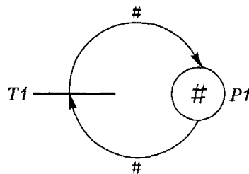
Рис. 3.16. Конструкція циклу
