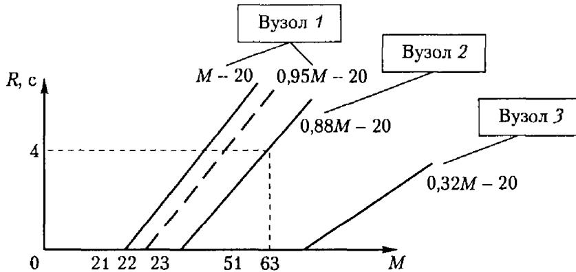
Рис. 2.24. Графіки для середнього часу обслуговування вимог
