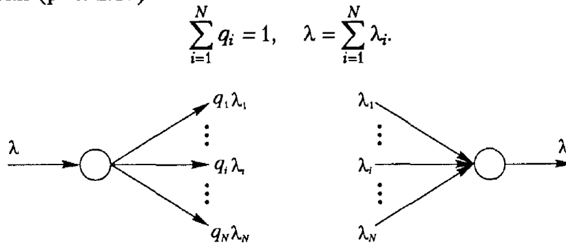
Рис. 2.17. Розгалуження та підсумовування потоків вимог вузла мережі
